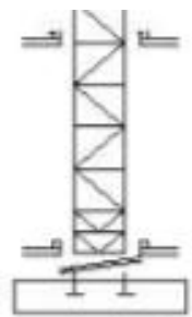
内爬式 Inner-climbing type
